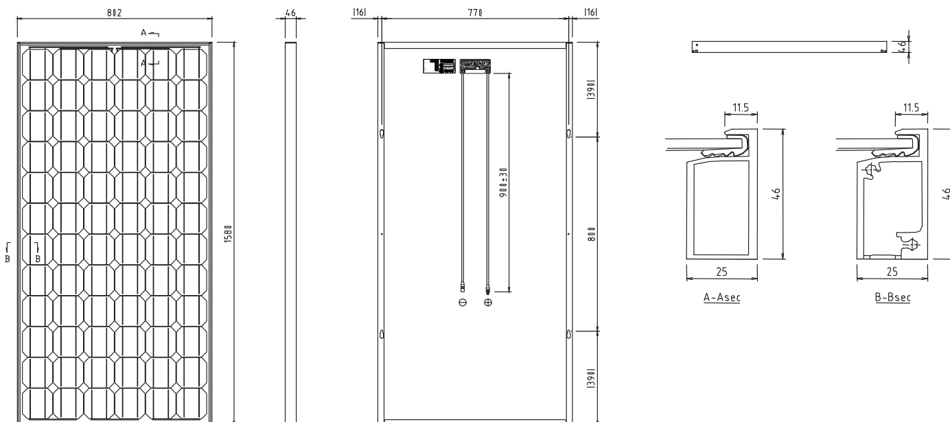
Vista posterior
